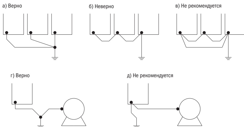
Рисунок 18 – Подключение контура заземления
