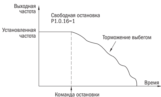
Рисунок 56 – Остановка выбегом
