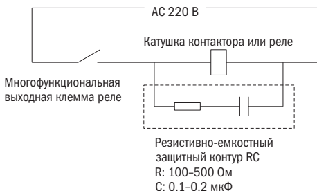
Рисунок 16 – Подключение выходного реле на переменный ток
