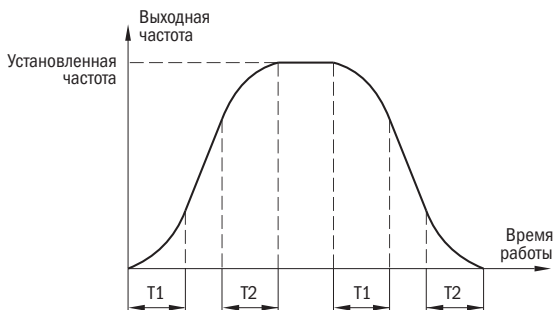
Рисунок 27 – Соотношение S-кривых
