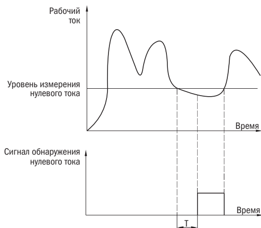
Рисунок 37 – Измерение нулевого тока
