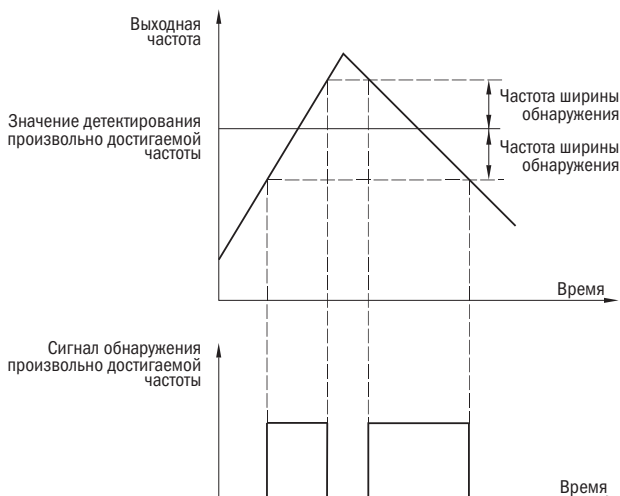
Рисунок 36 – Произвольно достигаемая частота
