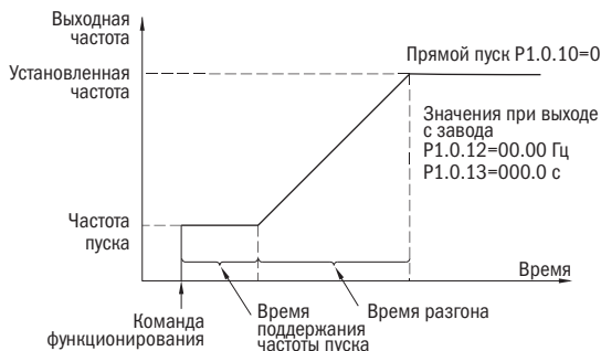
Рисунок 52 – Прямой пуск
