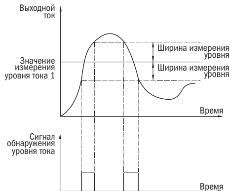
Рисунок 39 – Измерение уровня тока
