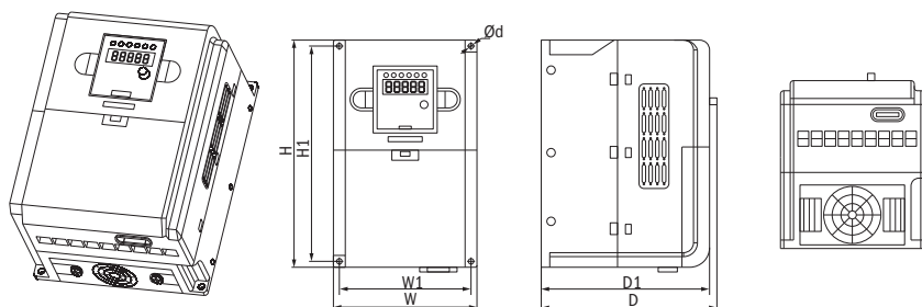
Рисунок 3 – Размеры габарита 2
