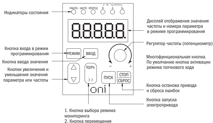
Рисунок 19 – Пульт управления преобразователя частоты
