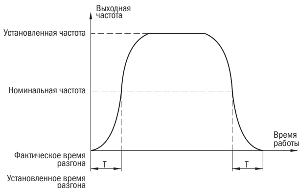
Рисунок 26 – S-кривая ускорения и замедления
