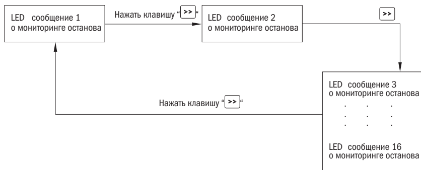
Рисунок 21 – Алгоритм просмотра состояния преобразователя частоты
