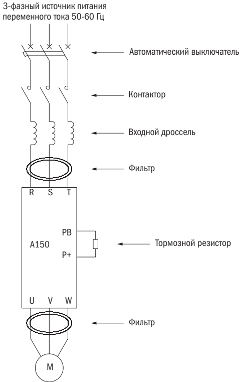
Рисунок 7 – Подключение периферийных устройств
