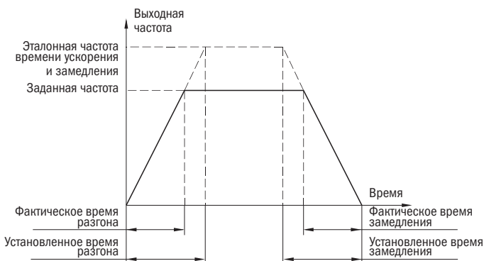
Рисунок 25 – Время ускорения и замедления
