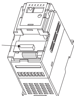
Рисунок В.8 – Место подключения платы расширения
