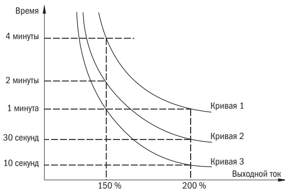
Рисунок 31 – Кривые защиты от перегрузки
