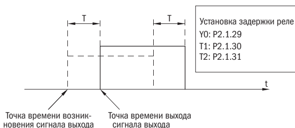
Рисунок 63 – Задержка срабатывания выходного реле
