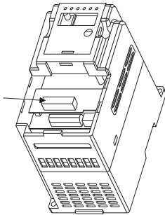
Рисунок В.4 – Место подключения платы расширения
