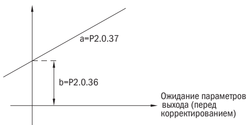
Рисунок 61 – Настройка аналогового выхода
