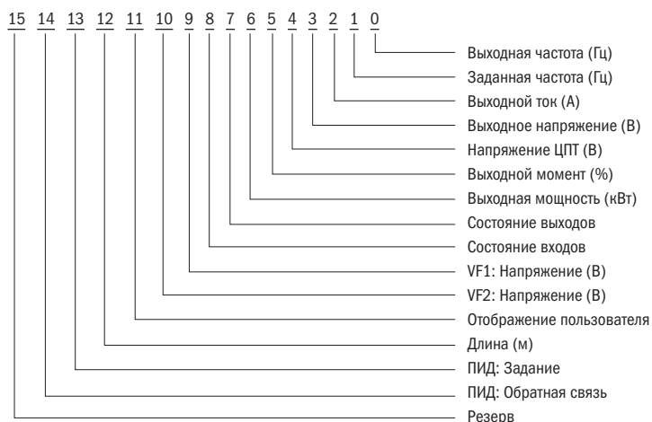
Рисунок 42 – Отображение 1 LED при работе
