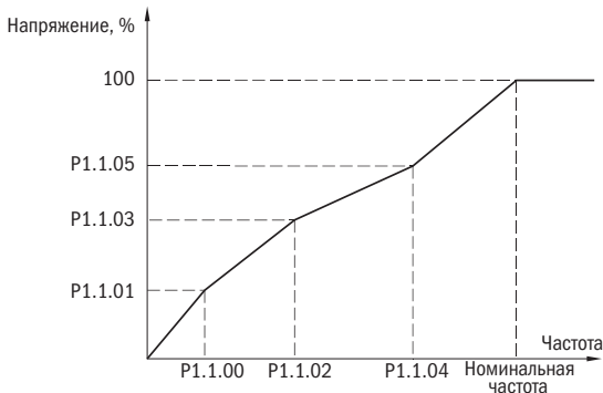
Рисунок 32 – Произвольная кривая V/F
