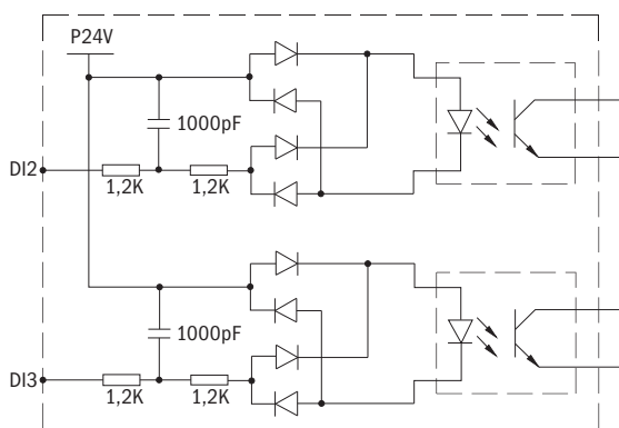
Рисунок 14 – Схема цифровых входов
