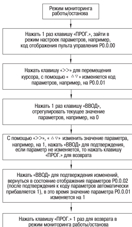
Рисунок 23 – Настройка параметров с помощью пульта управления
