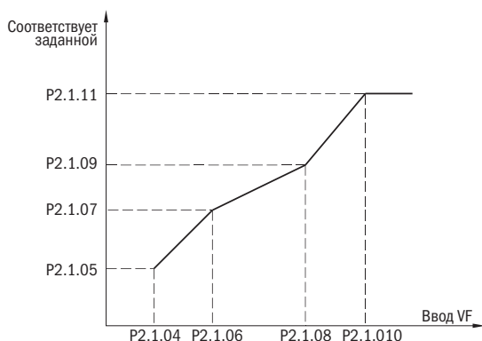
Рисунок 33 – Произвольная кривая 3 аналогового входа
