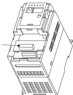
Рисунок В.2 – Место подключения платы расширения
