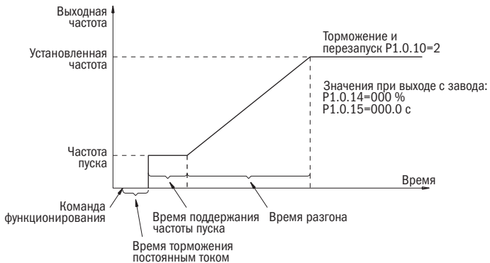
Рисунок 54 – Пуск с торможением постоянным током
