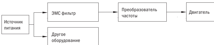
Рисунок 11 – Подключение фильтра со стороны входа
