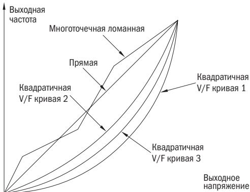
Рисунок 29 – V/F-кривые
