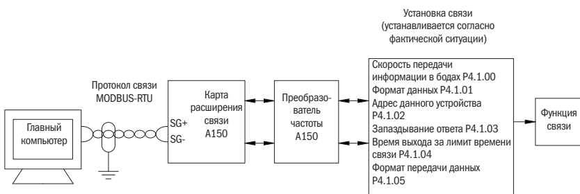
Рисунок 64 – Соединение по интерфейсу с внешним PLC
