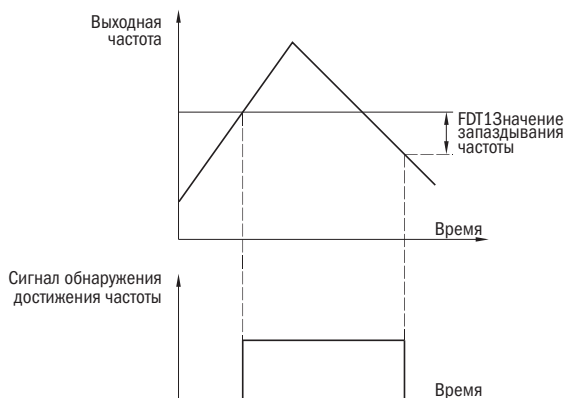
Рисунок 35 – Измерение частоты FDT1
