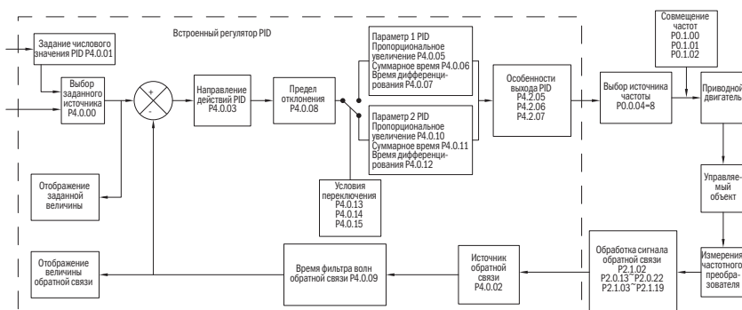
Рисунок 59 – Структура ПИД-регулятора
