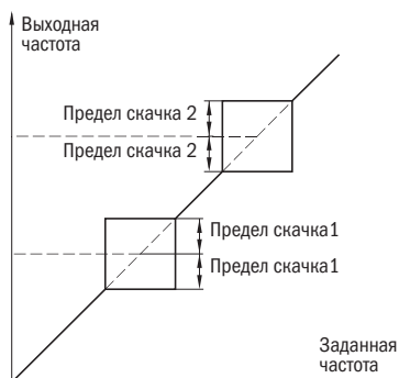
Рисунок 28 – Скачкообразные частоты
