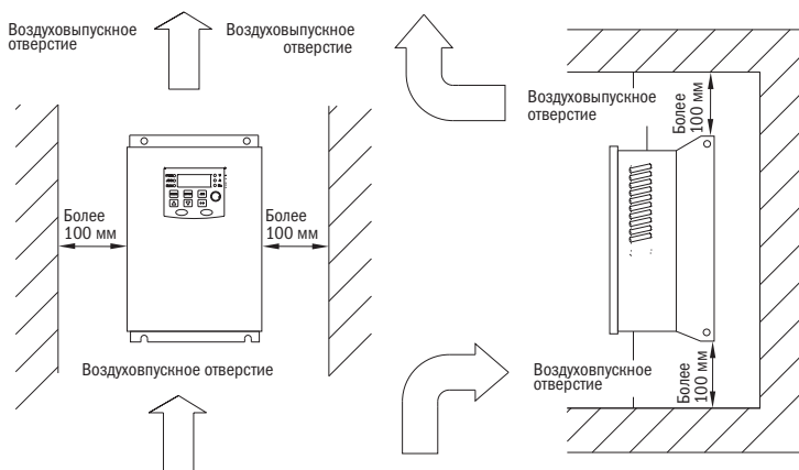
Рисунок 6 – Способ установки преобразователя частоты
