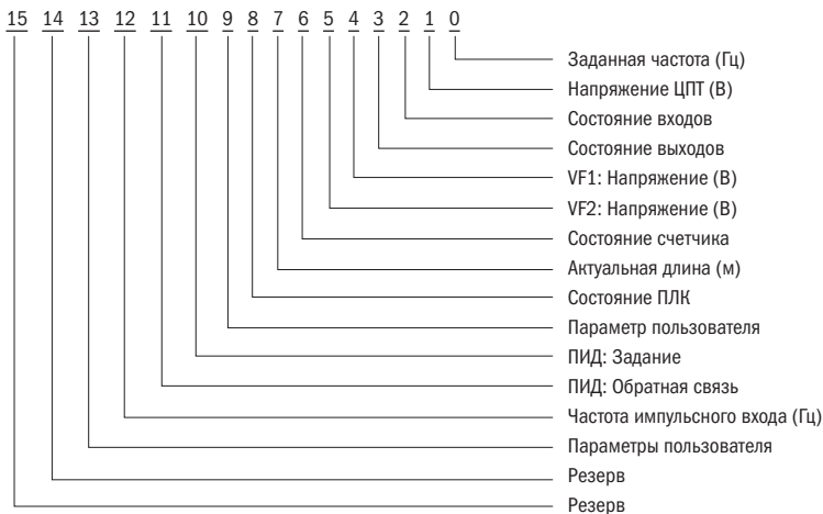
Рисунок 44 – Отображение LED при остановке
