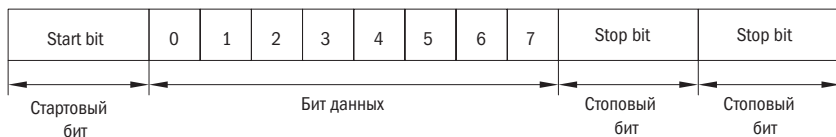
Рисунок 66 - 8-N-2, P4.1.01 = 0
