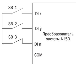
Рисунок 50 – Трехпроводной способ управления 1
