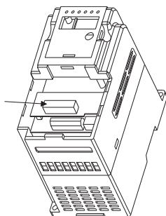
Рисунок В.6 – Место подключения платы расширения
