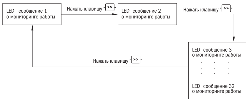
Рисунок 22 – Просмотр состояния преобразователя в остановленном состоянии
