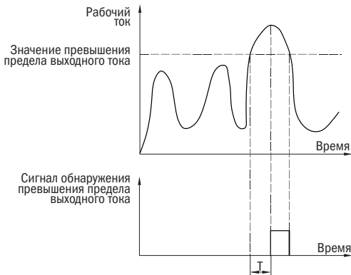
Рисунок 38 – Измерение превышения выходного тока
