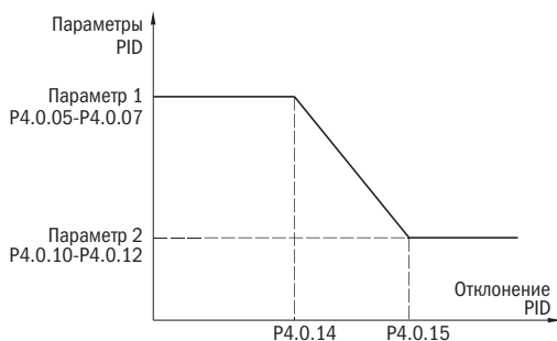
Рисунок 40 – Переключение ПИД
