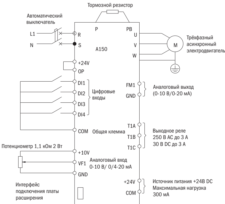
Рисунок 12 – Клеммная колодка платы управления преобразователя
