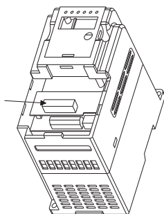
Рисунок В.3 – Место подключения платы расширения
