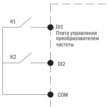
Рисунок 15 – Схема подключения цифровых входов
