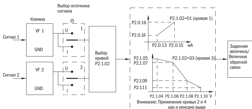
Рисунок 60 – Настройка аналоговых входов
