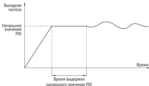
Рисунок 41 – Начальное значение ПИД
