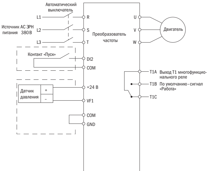
Рисунок 65 – Схема подключения преобразователя частоты для поддержания давления с датчиком 4–20 мА
