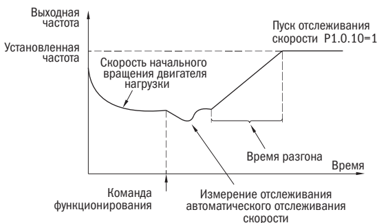
Рисунок 53 – Пуск с поиском скорости
