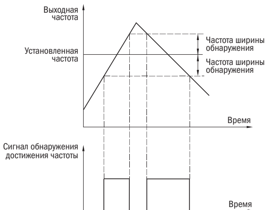
Рисунок 34 – Ширина обнаружения заданной частоты
