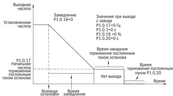
Рисунок 55 – Остановка замедлением
