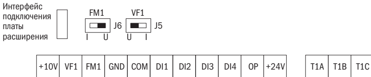
Рисунок 12 – Клеммная колодка платы управления преобразователя
