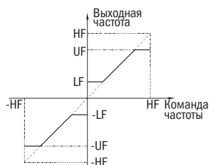
Рисунок 24 – Пределы частоты
