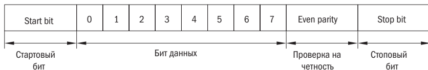
Рисунок 67 - 8-E-1, P4.1.01 = 1
