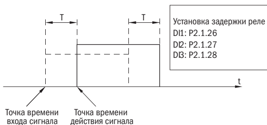
Рисунок 62 – Задержка срабатывания времени T
