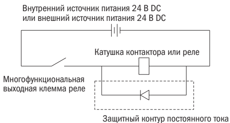
Рисунок 17 – Схема подключения выходного реле на постоянный ток
