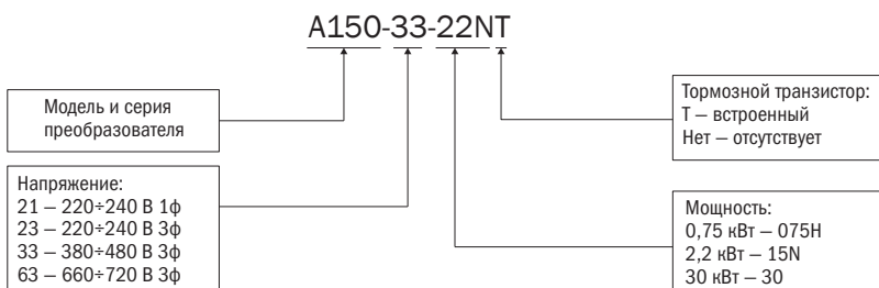
Рисунок 1 – Пример расшифровки артикула преобразователя частоты
