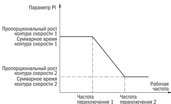
Рисунок 30 – Частоты переключения
