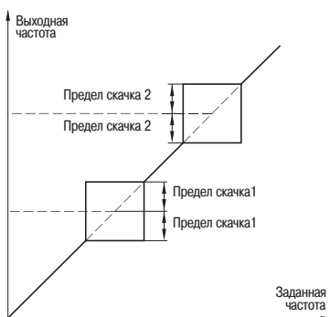
Рисунок 29 — Скачкообразные частоты
