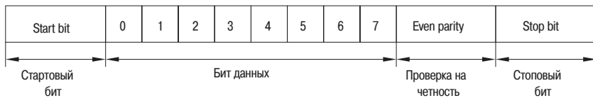
Рисунок 84 – 8-E-1, P4.1.01 = 1
