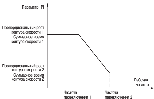
Рисунок 31 — Частоты переключения
