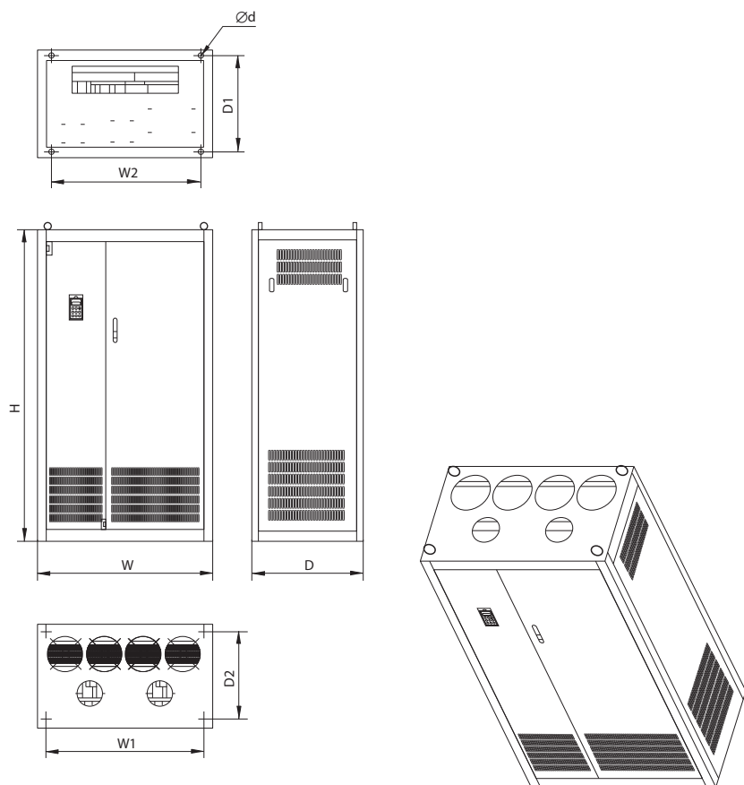
Габарит 5.8
