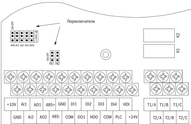
Рисунок 3.22 — Расположение клемм платы управления K750
