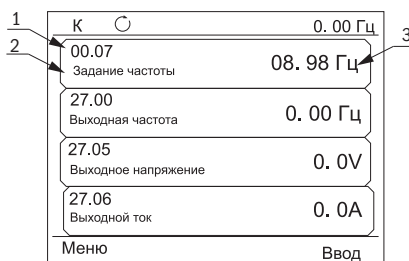
Рисунок 4.16 – Выбор параметра монитора состояния
