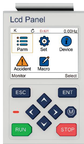
Рисунок 4.18 – Внешний вид LCD-пульта управления RCP-K750-LCD
