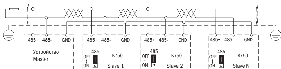
Рисунок 3.28 — Подключение нескольких преобразователей K750 в промышленную сеть с управлением от внешнего ПЛК
